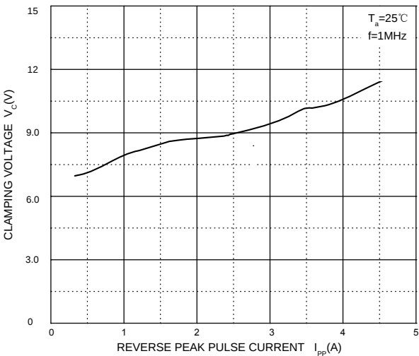
V_C ---- I_{PP}
