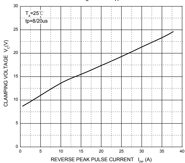
V_C — I_{PP}
