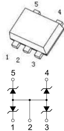
SOT-553
