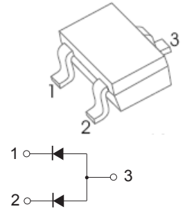
SOT-323
