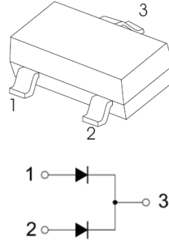
SOT-23
