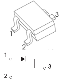
SOT-323
