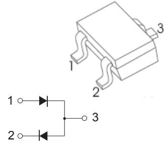
SOT-323
