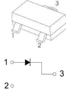
SOT-23
