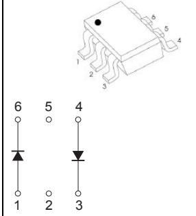
SOT-363
